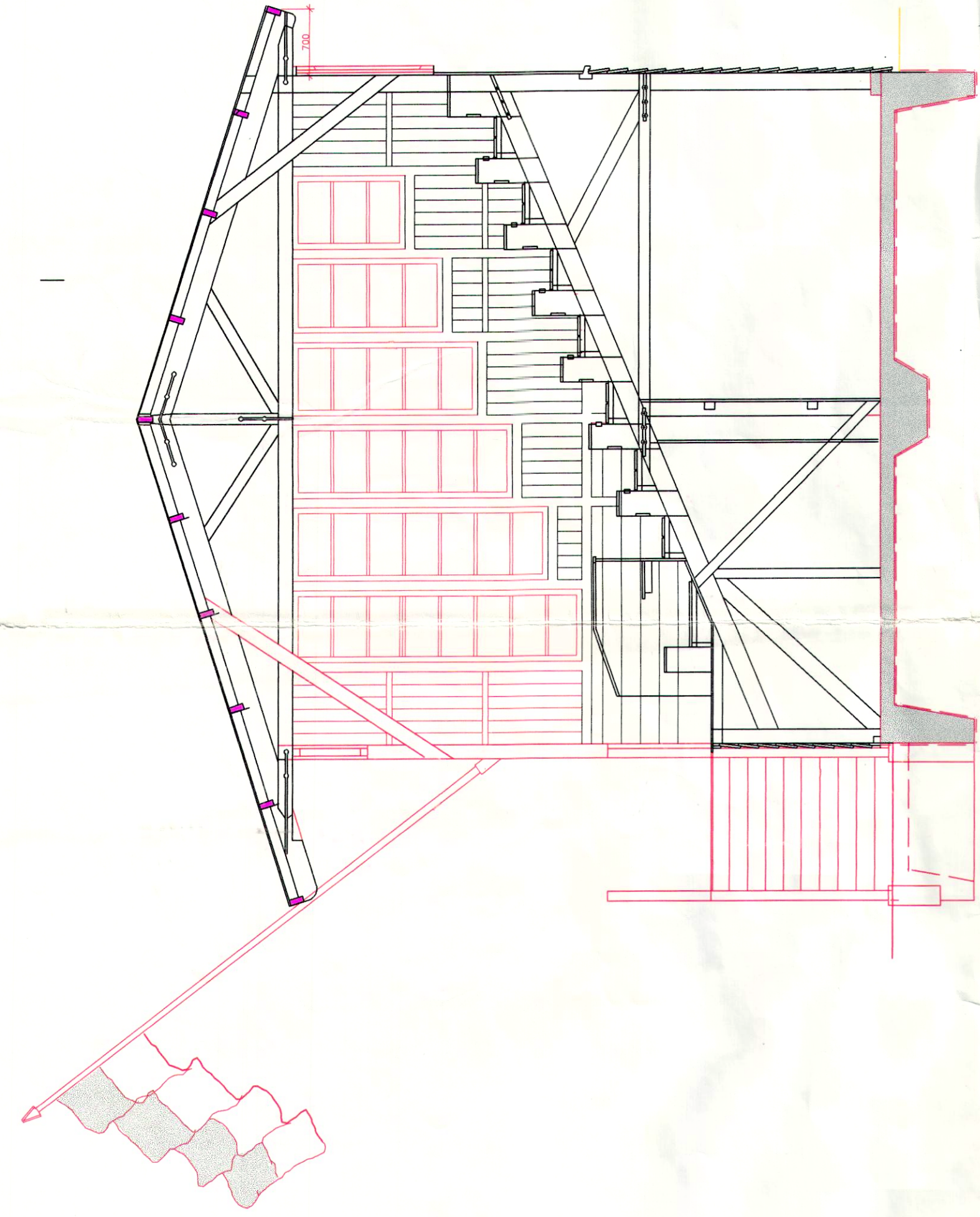
doorsnede A-A
